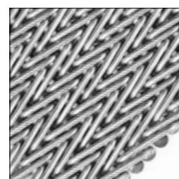
Runddrahtgliedergurte mehrfach geflochten Gruppe 4000
