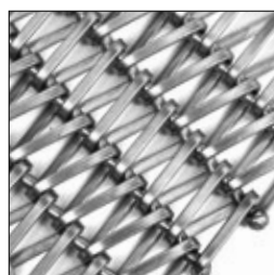
Flachdrahtgliedergurte Gruppe 300
