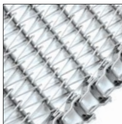
Kurvengängige Fördergurte Gruppe 400 RW
